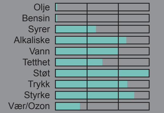
Naturgummi (NR)
