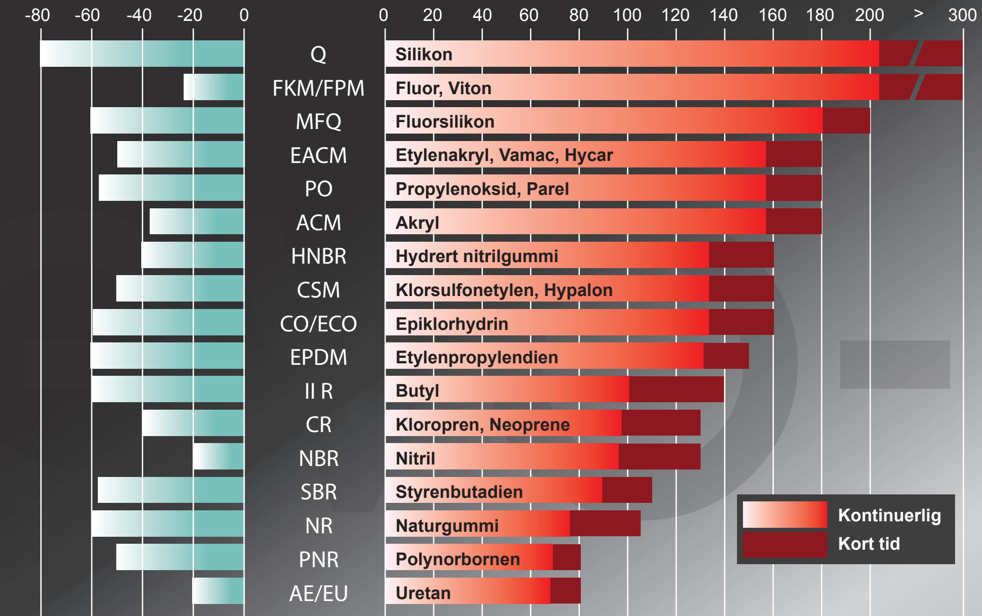
LAVESTE OG HØYESTE DRIFTSTEMPERATUR
