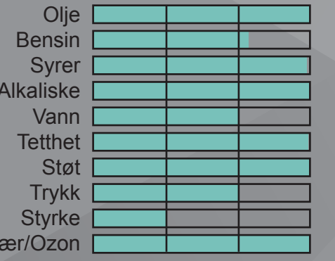
Epiklorhydrin (CO/ECO)
