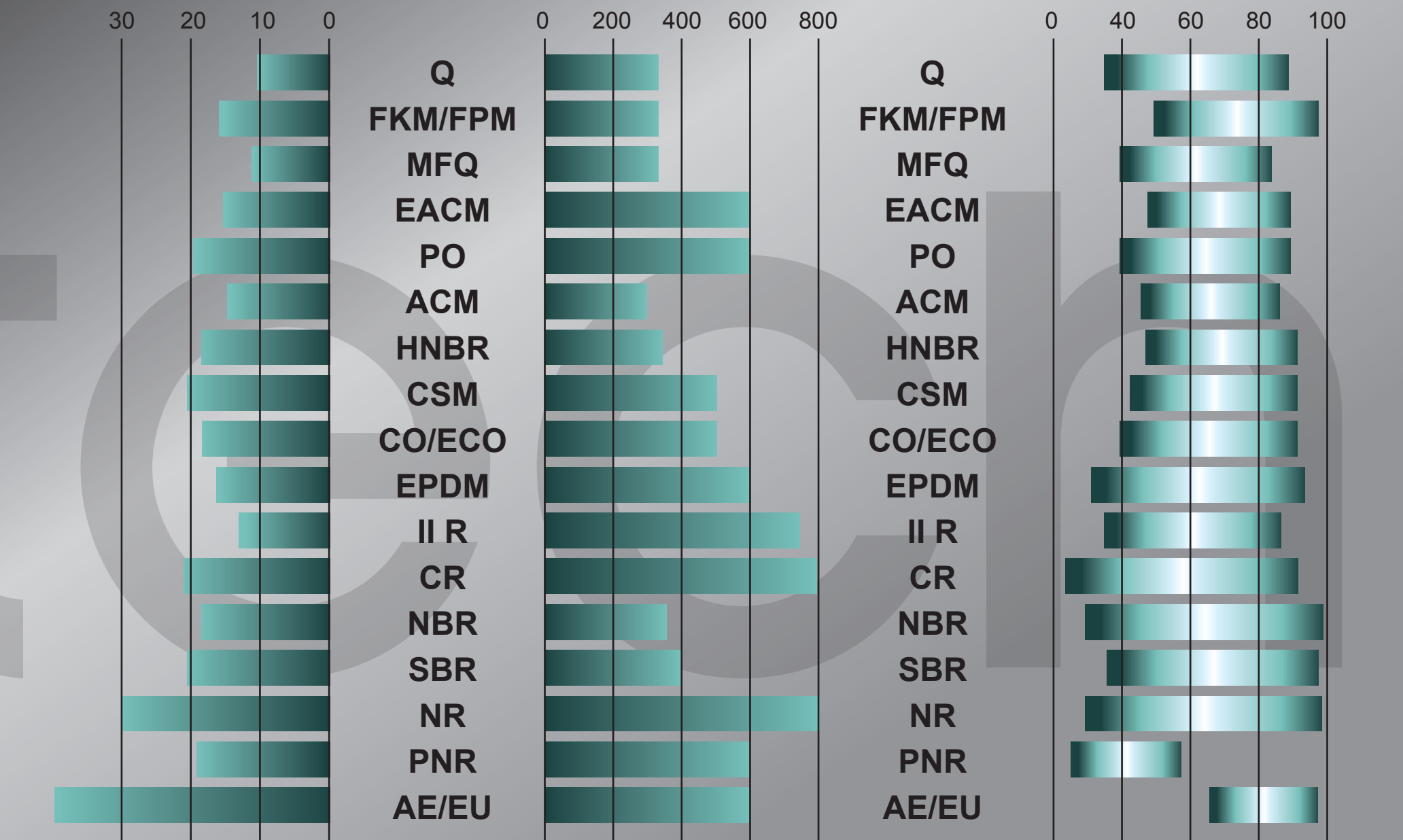
STREKKFASTHET MPa
