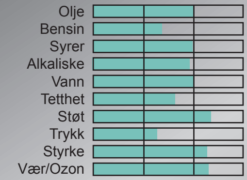
Neoprene (CR)
